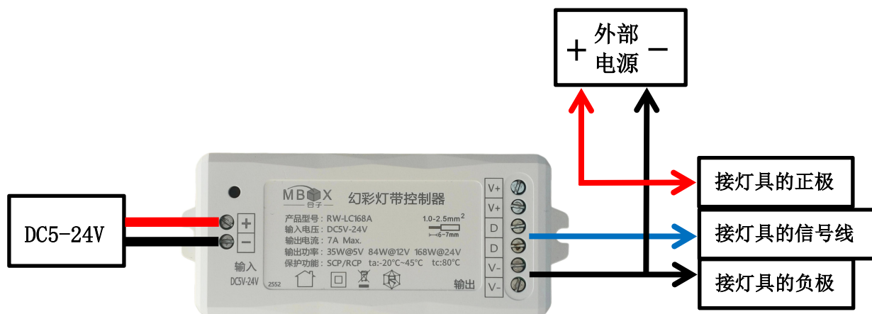
RW-LC168A 接 “外部电源+” “外部电源-” “输出 D” “输出 V-”
